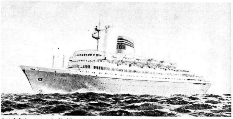
Amerikalinjens nye cruiseskip blir praktisk talt søsterskip av M/S «Sagafjord», men 1 000 br.tonn større. Det blir 625 fot langt og bredden blir 82 fot. Innredningsmessig blir det også enkelte forandringer.
